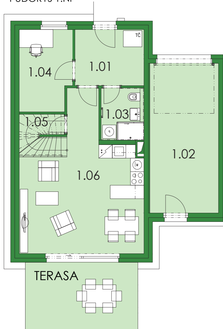
PŮDORYS 1.NP
